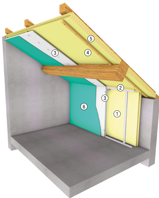
Schéma N°10 Combles aménageables : isolation avec parement rapporté
